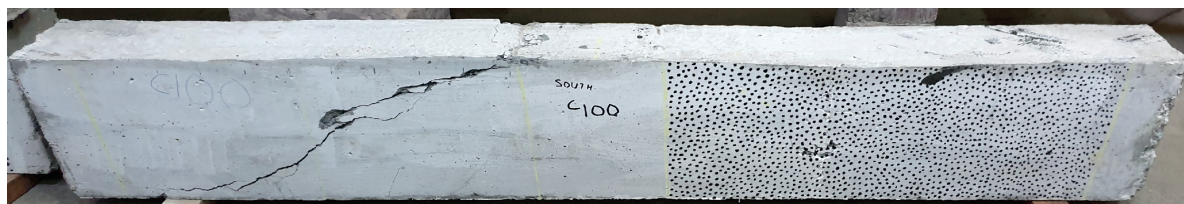
a) C100 Wzorec pęknięcia belki - zniszczenie przez ścinanie a) C100 Beam crack pattern at ultimate – failed in shear
