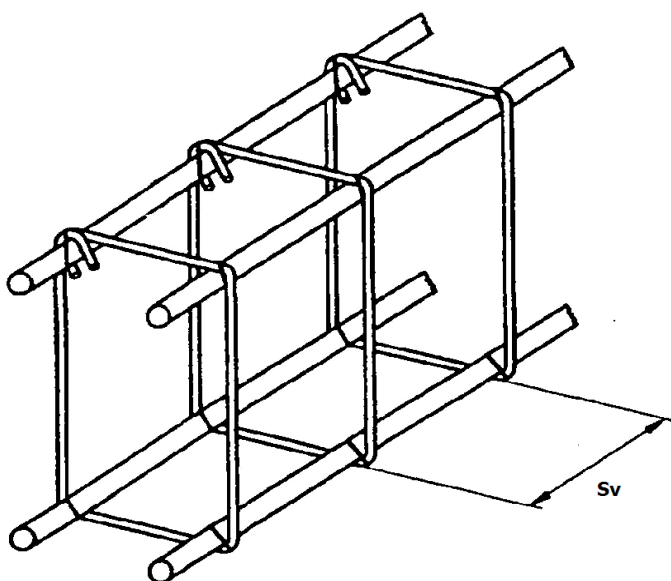
Rys. 2. Zbrojenie z konwencjonalnymi strzemionami
