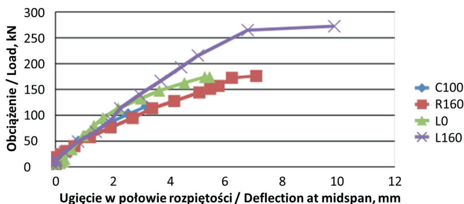
Rys. 6. Zależność obciążenia-przemieszczenia
