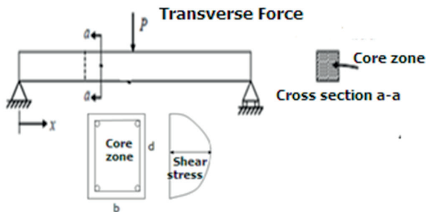
Rys. 1. Rozkład naprężeń tnących w przekroju prostokątnym
