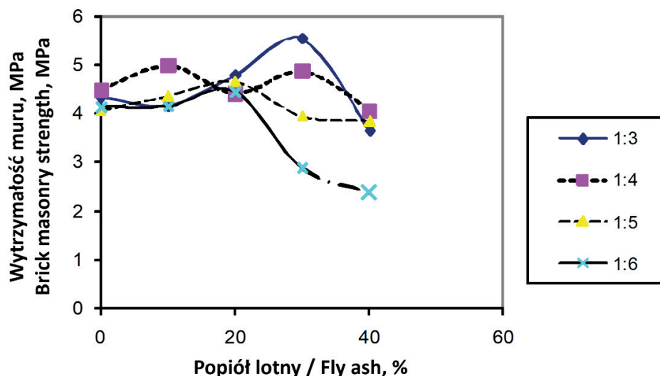
Rys. 3. Zależność wytrzymałości na ściskanie muru od zawartości popiołu lotnego [wytrzymałość cegieł: 11,31 MPa]
