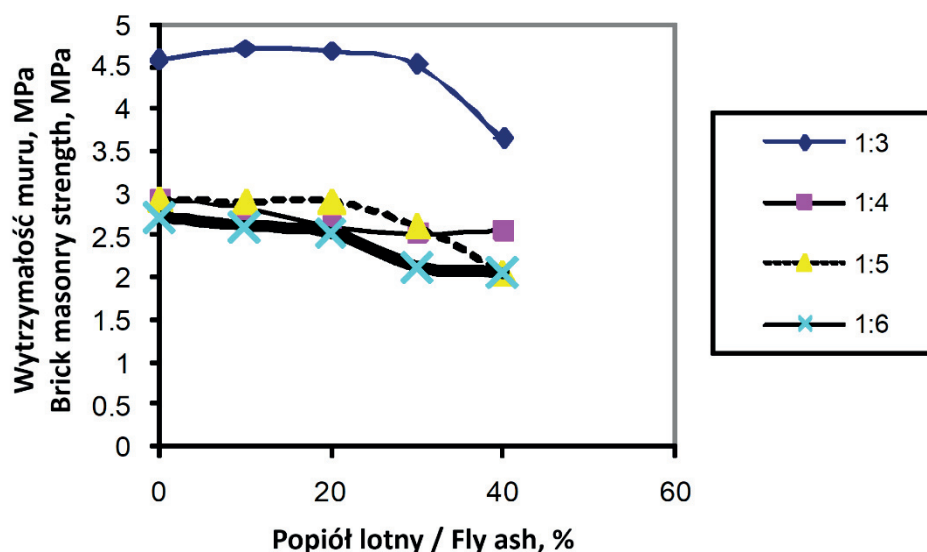
Rys. 2. Zależność wytrzymałości na ściskanie muru od zawartości popiołu lotnego [wytrzymałość cegieł: 3,37 MPa]
