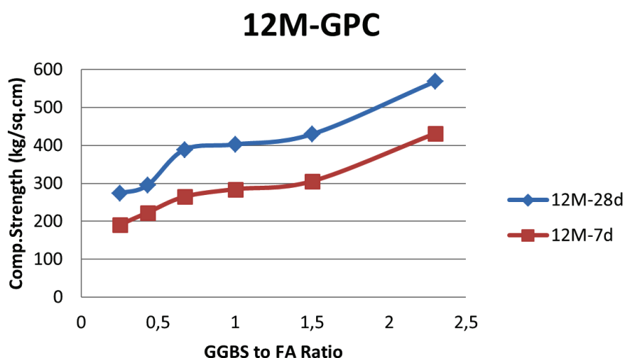
Rys. 4. Wpływ stosunku żużel/popiół na wytrzymałość na ściskanie GPC, 12 moli/L
