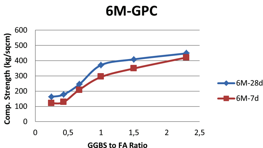
Rys. 1. Wpływ stosunku żużel/popioł na wytrzymałość na ściskanie GPC, 6 moli/L
