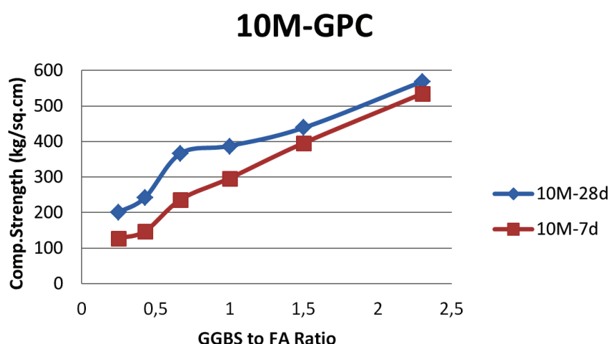
Rys. 3. Wpływ stosunku żużel/popiół na wytrzymałość na ściskanie GPC, 10 moli/L
