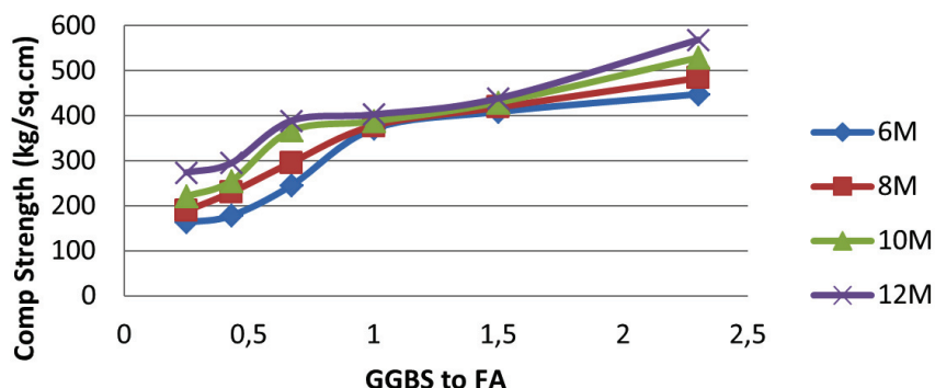
Rys. 5. Wpływ stosunku żużel/popioł na wytrzymałość na ściskanie GPC
