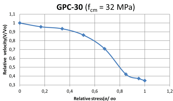
Rys. 4. Zmiany szybkości rozchodzenia się fali ultradźwiękowej w betonie bez klinkieru klasy \approx C25/30
