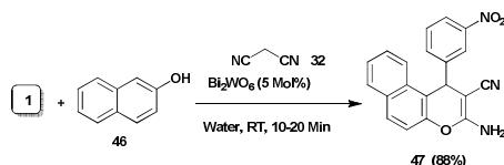
Scheme-4. 2-amino-4H-benzo[b]pyran (47)
