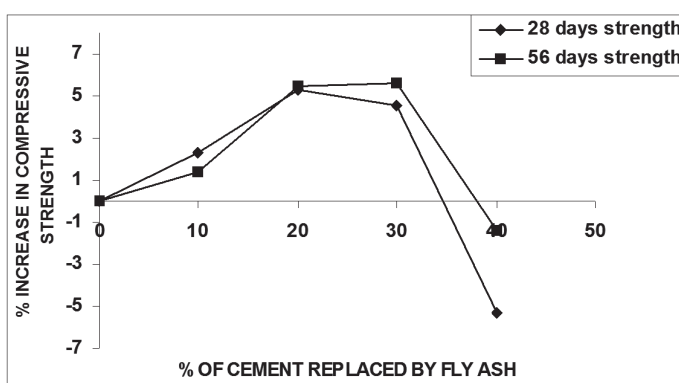
Rys. 8. % wzrostu wytrzymałości na ściskanie betonu w zależności od ilości cement zastąpionego popiołem lotnym w przypadku zastąpienia 8% pyłem krzemionkowym
