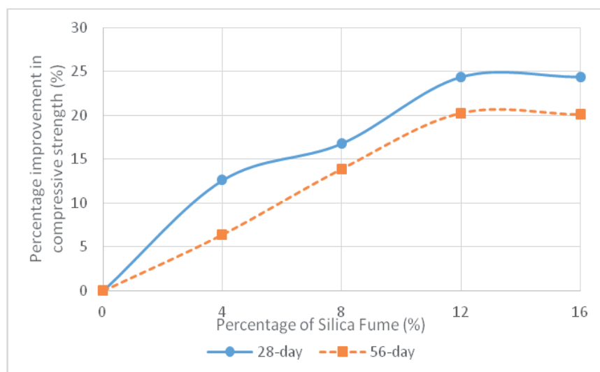
Rys. 14. Poprawa wytrzymałości betonu w zależności od dodatku pyłu krzemionkowego zastępującego cement w przypadku jego równoczesnego zastąpienia przez 20% popiołu lotnego
