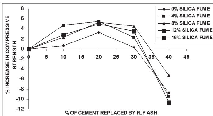
Rys. 13. % wzrostu wytrzymałości betonu na ściskanie w zależności od ilości cementu zastąpionego popiołem lotnym w przypadku różnego dodatku pyłu krzemionkowego również zastępującego cement
