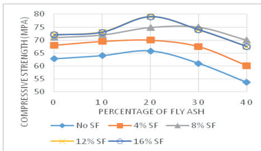
Rys. 12. Zbiorcze zestawienie wytrzymałości betonu po 56 dniach
