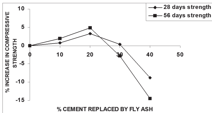
Rys. 6. % wzrostu wytrzymałości na ściskanie betonu w zależności od ilości cement zastąpionego popiołem lotnym
