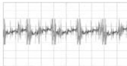
(d) Voltage: 0.5 V/div., Time: 5 \mu secs./div., PRF = 100 kHz
