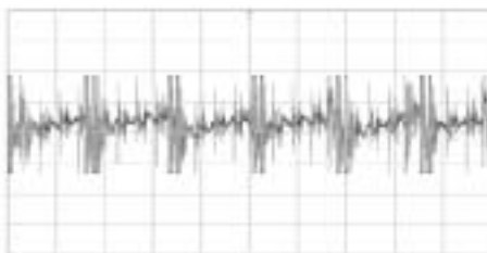
(e) Voltage: 0.5 V/div., Time: 5 \mu secs./div., PRF = 115 kHz
